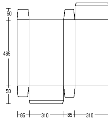
[그림8-3] 냉동오징어 8kg 포장 설계도
