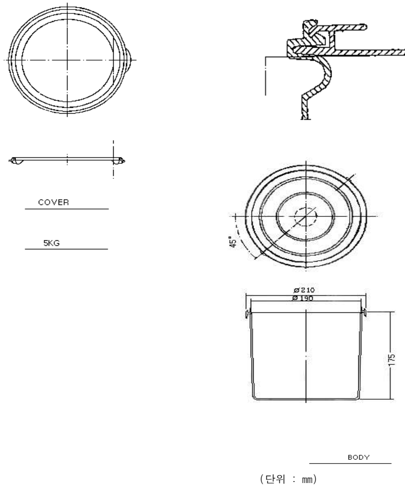
[그림7-3]새우젓, 멸치젓 5kg 포장 설계도
