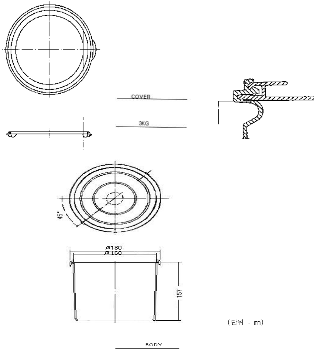
[그림 7-2] 새우젓, 멸치젓 3kg 포장 설계도
