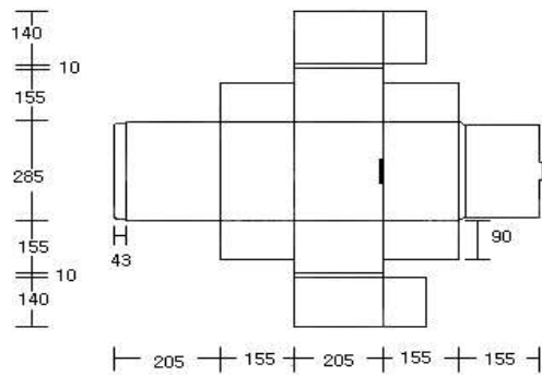
[그림9-5] 간미역 5kg 포장 설계도
