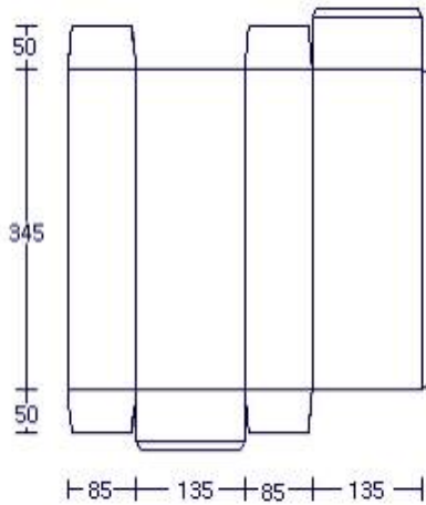
[그림8-1] 냉동오징어 2kg 포장 설계도
