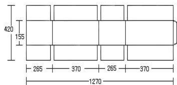
[그림9-6] 간미역 10kg 포장 설계도
