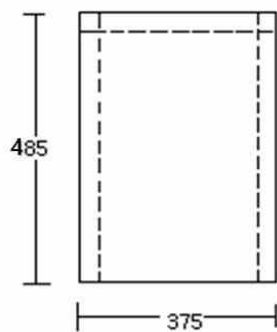
[그림2-3] 바지락 10kg 포장 설계도
