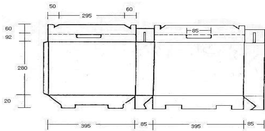
[그림5] 굴비 10마리 포장 설계도
