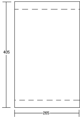
[그림3-2] 꼬막 5kg 포장 설계도
