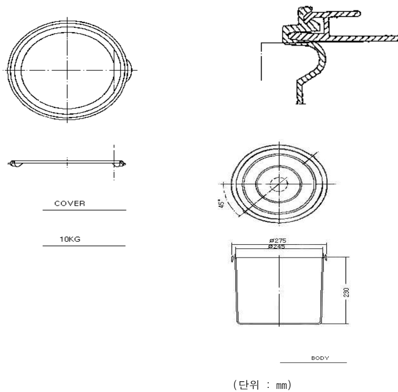
[그림7-4]새우젓, 멸치젓 10kg 포장 설계도
