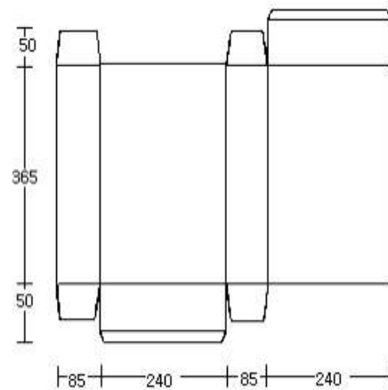
[그림8-2] 냉동오징어 4kg 포장 설계도
