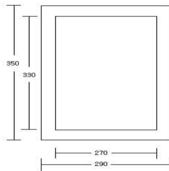
[그림9-3] 간미역 1kg 포장 설계도
