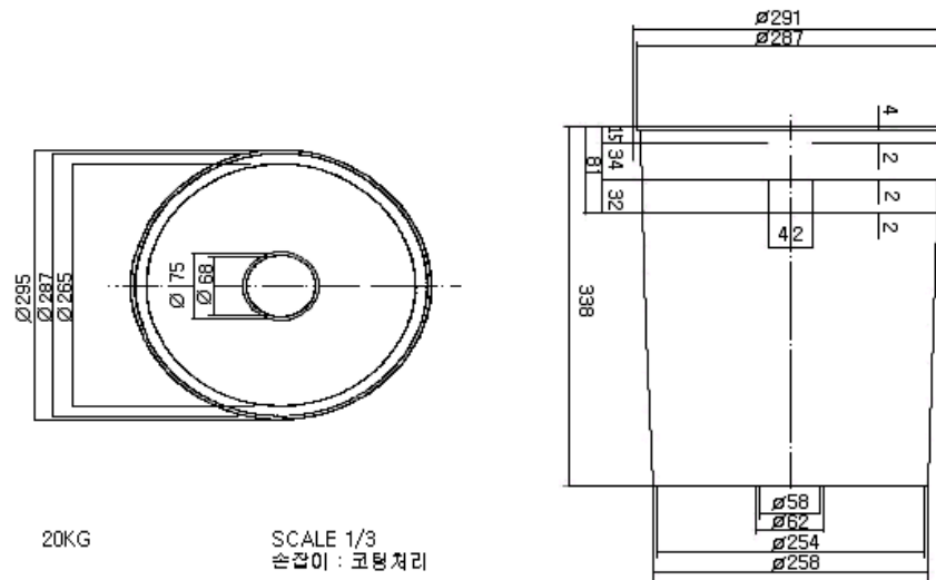
[그림7-5] 멸치젓 20kg 포장 설계도
