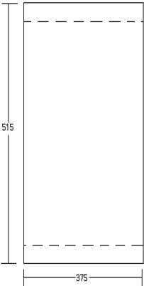
[그림3-3] 꼬막 10kg 포장 설계도
