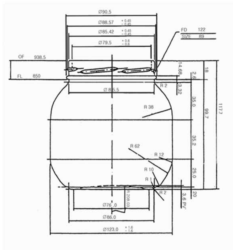
[그림 7-1] 새우젓, 멸치젓 1kg 포장 설계도
