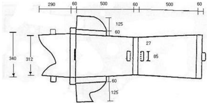
[그림4] 북어 10마리 포장 설계도
